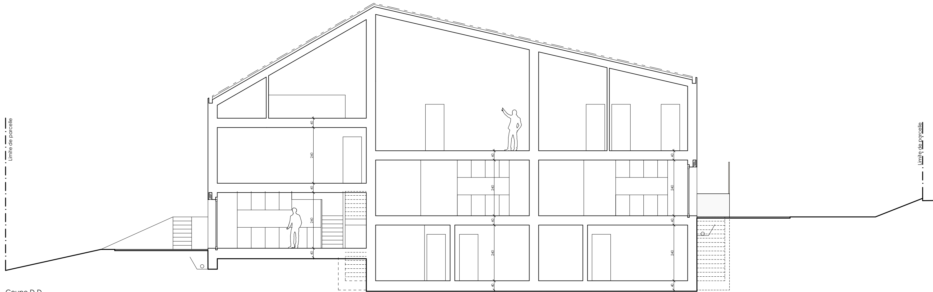
Coupe D-D
